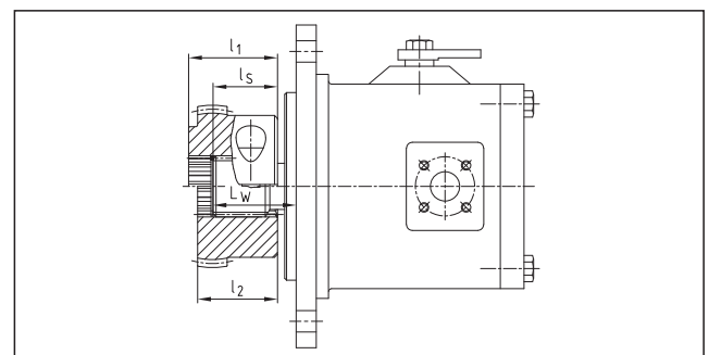
piasta zaciskowa
